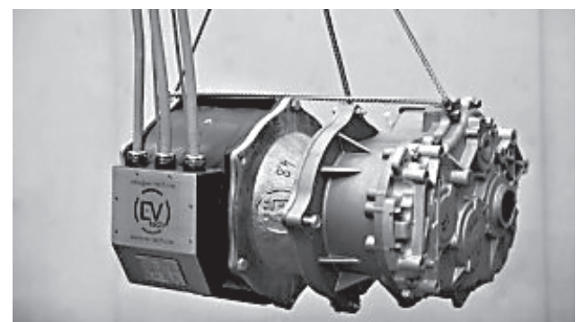
Вентильно-индукторный электродвигатель
